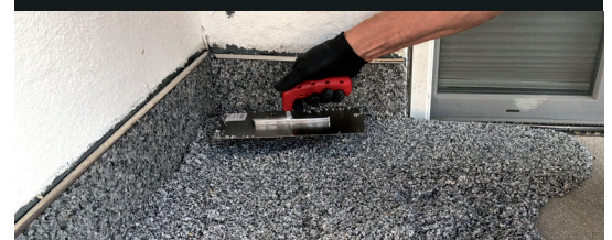
5. Aufbringen des Granulatgemisches ALSAN 817 Bindemittel / ALSAN 887 Marmorkiesel
